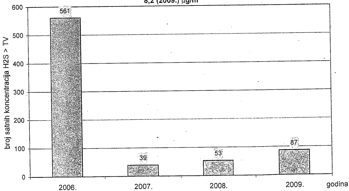
Sisak: grafikon satnih koncentracija H_2S > 10 (2006.), 9,4 (2007.), 8,8 (2008.) i 8,2 (2009.) \mu g/m^3
