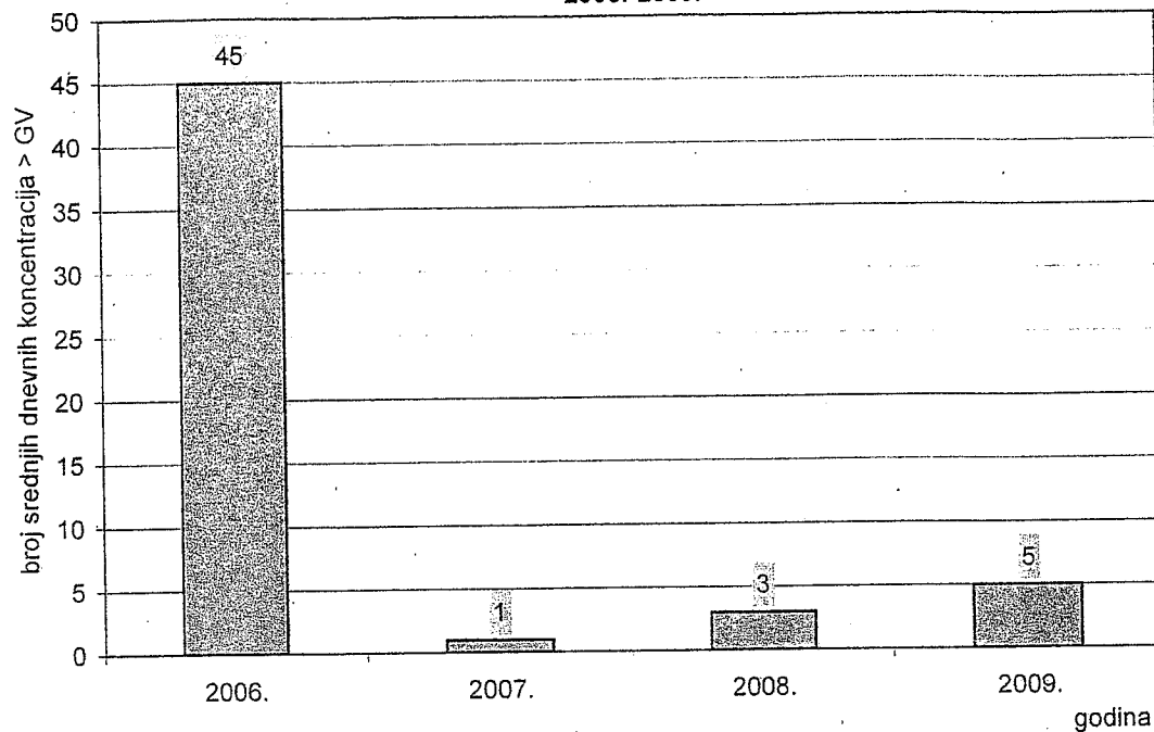
Sisak: grafikon srednjih dnevnih koncentracija H_2S > 5 \mu g/m^3 u periodu 2006.-2009.
